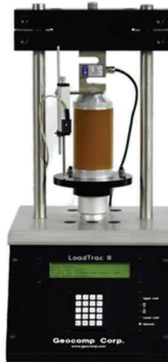
Sistema Standard para Compresión no Confinada Completamente Automatizado
